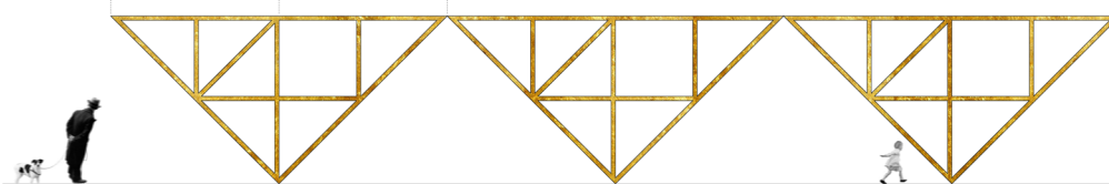
Estructura dels bastidors dels triangles invertits i revestiment de pa d'or E. 1:200 El revestiment de pa d'or esdevé un fenomen variable atenent a les condicions lluminiques i atmosfèriques
