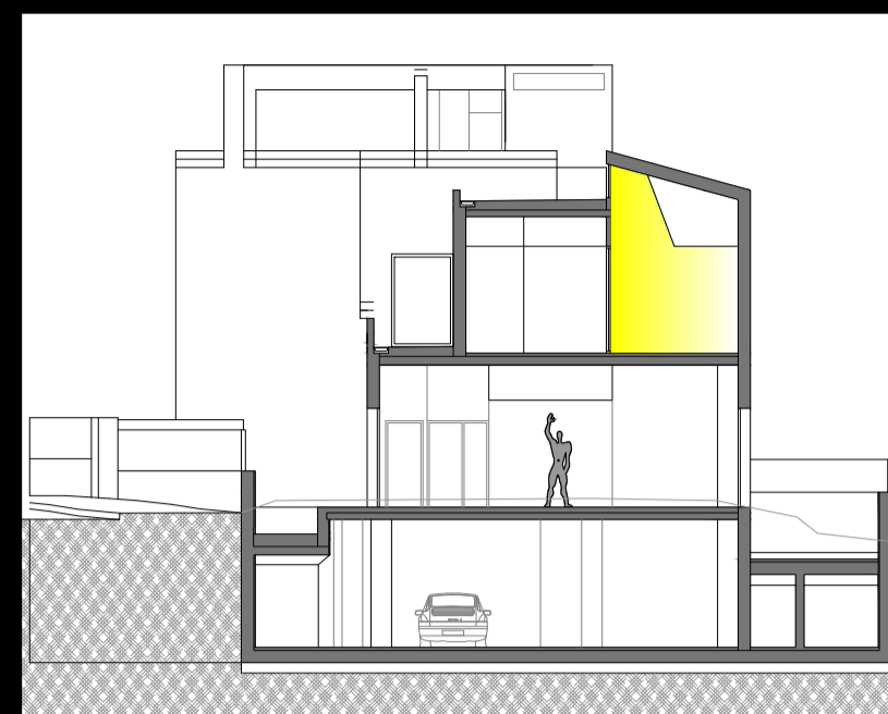
SECCIÓN A-A' E:1/200
