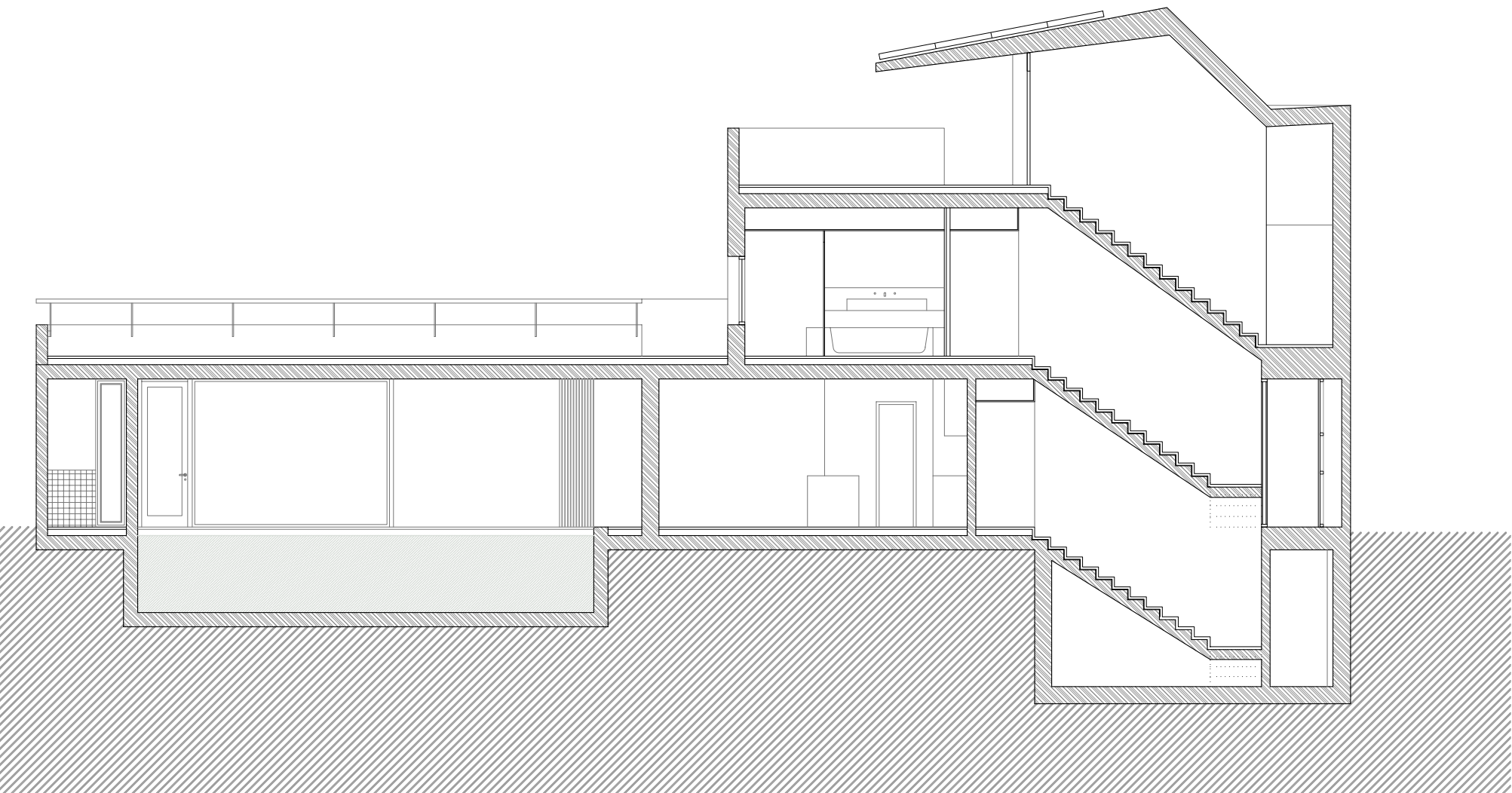
secció longitudinal piscina e: 1/100
