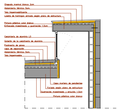
detalls secció
