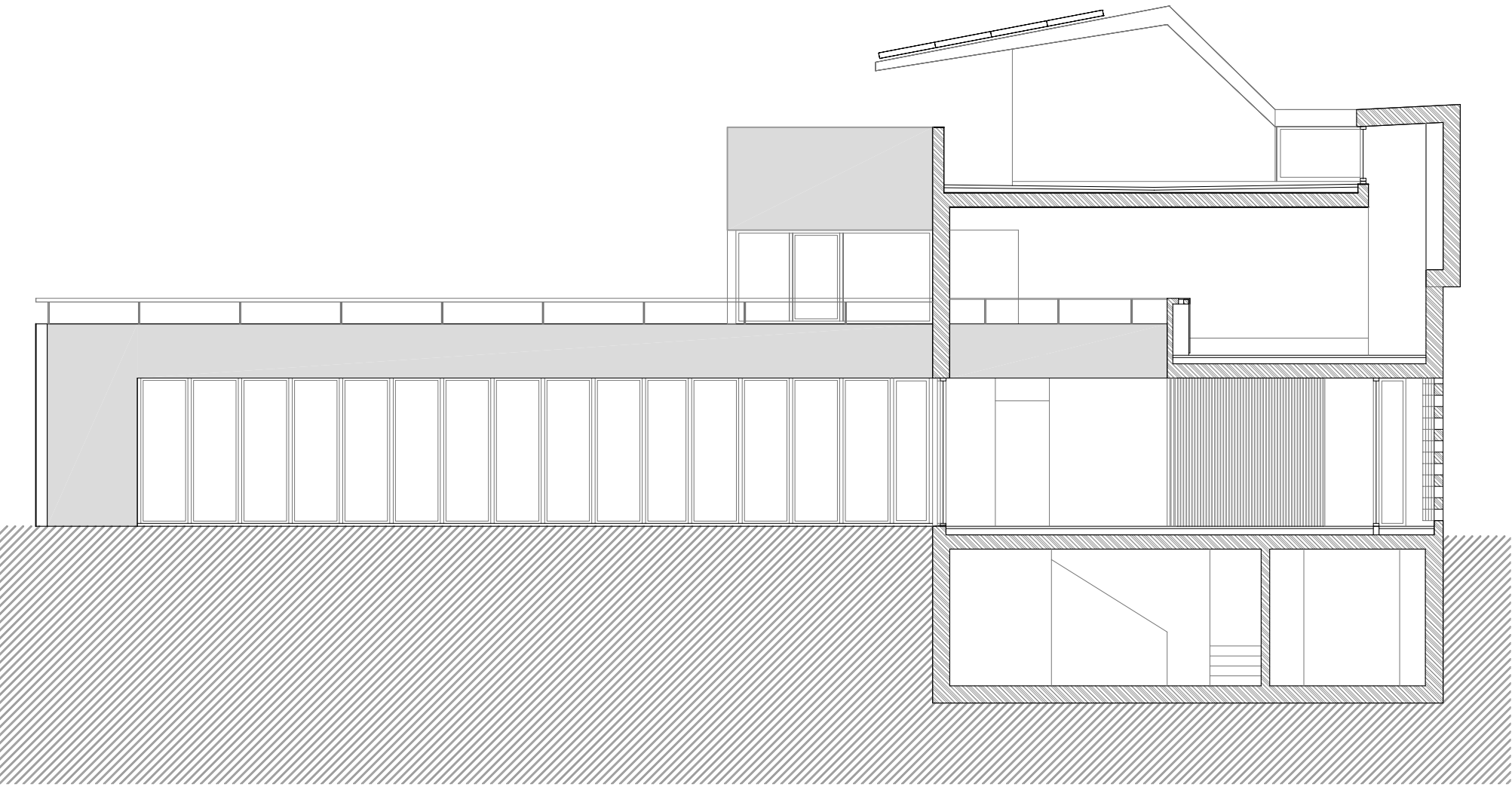
secció longitudinal lluernari e: 1/100
