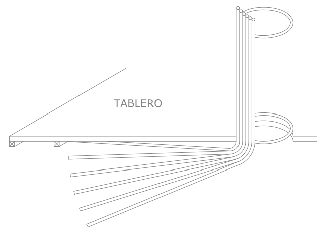
DETALLE BASE PILARES
