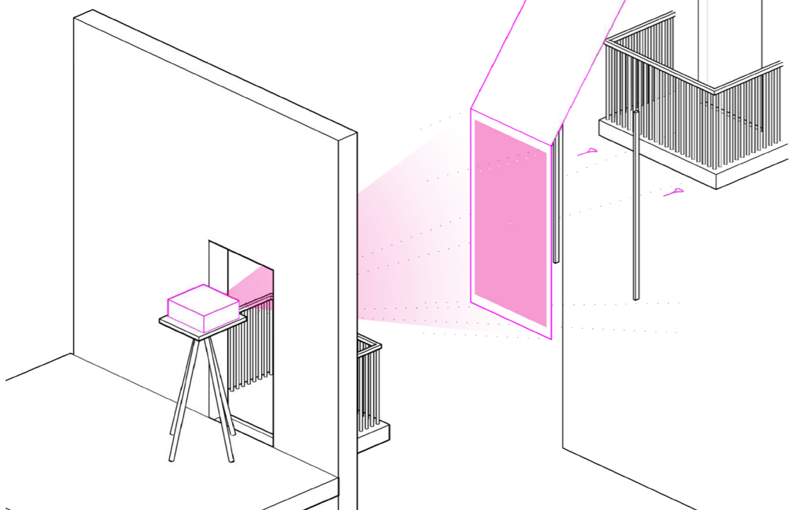
* axonometria detallent el sistema constructiu de la projecció
