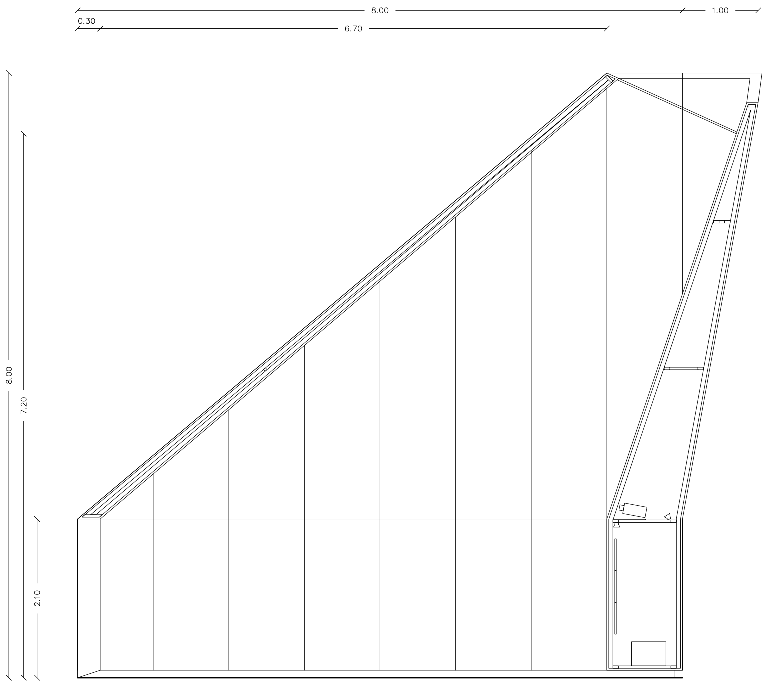
SECCIÓN POR EL ACCESO E 1:50
