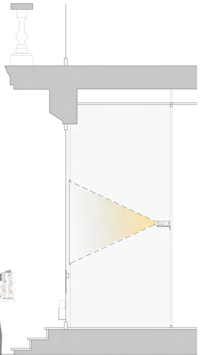
Secció Aparador E: 1/40
