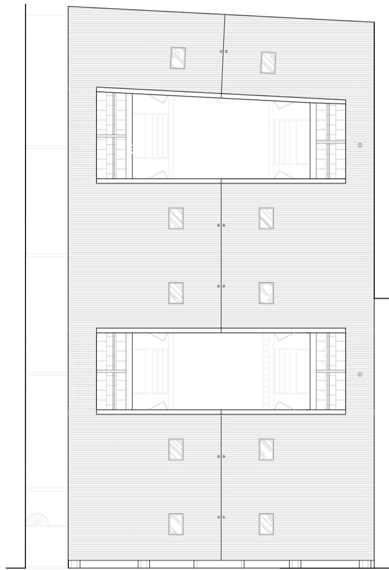
PLANTA COBERTA
