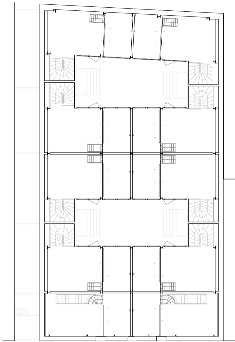
PLANTA ALTELL
