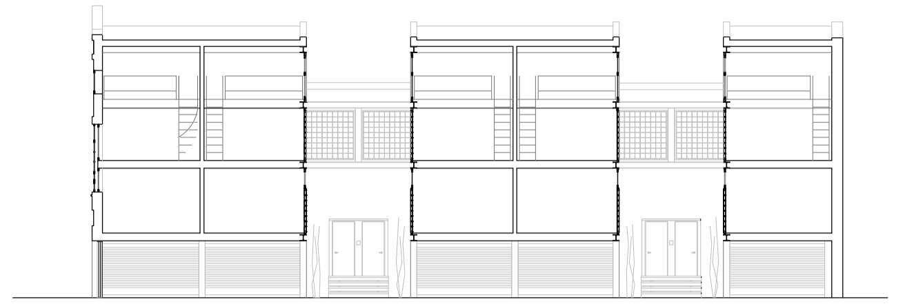
SECCIO CARRER
