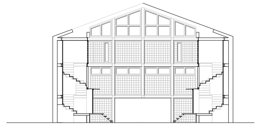
SECCIO PATI
